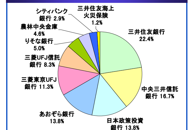
借入金の調達先分布 (2009年4月30日時点)
