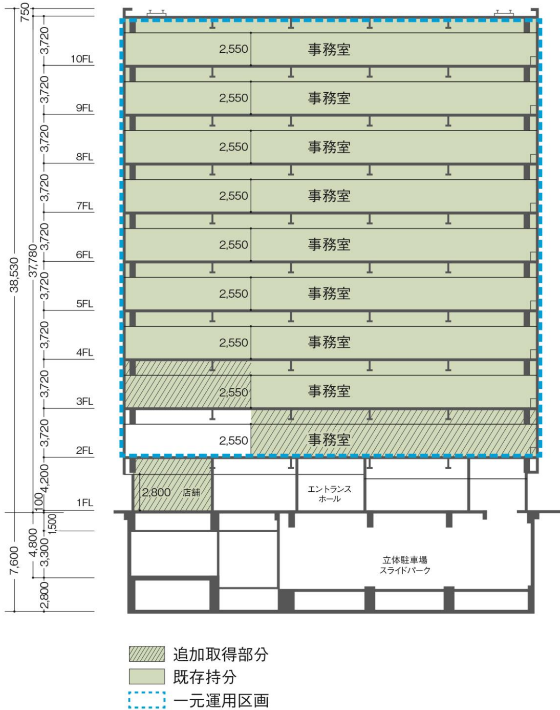
【参考資料 4】本物件の断面図
