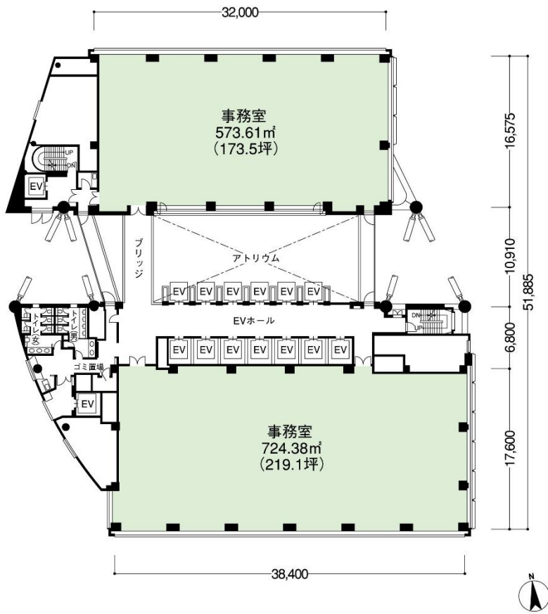
【参考資料3】本物件の基準階平面図(ツイン棟)
